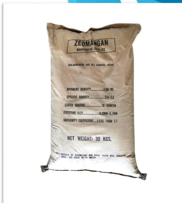
Zeomangan Manganese Zeolite
